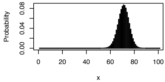
Bin(n=100, p=0.7)
