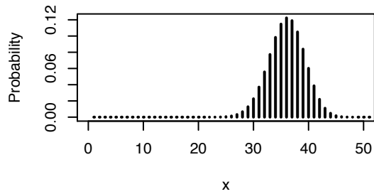
Bin(n=50, p=0.7)
