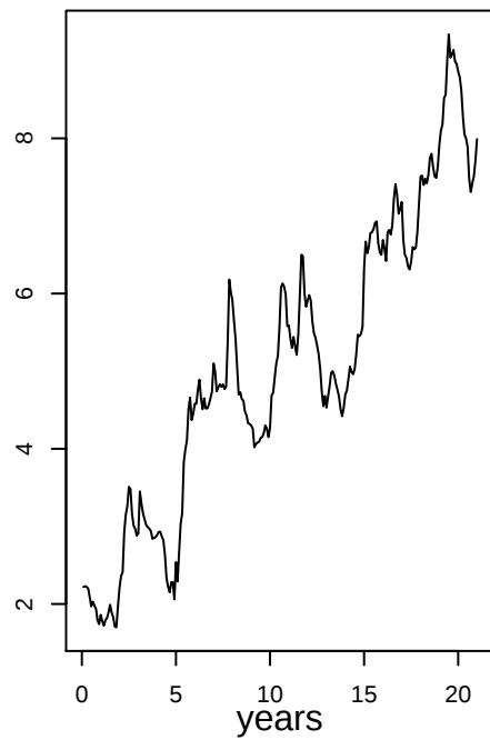
yield (data)
